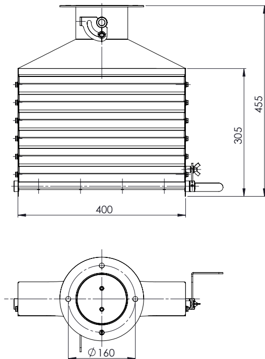
Hood For Manual Load Material : SUS Weight : 6.10 Kg. Unit : mm.
